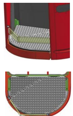
Die Grafiken zeigen Lage und Höhe der Lichtschranke (hellgrün), deren Unterbrechung die Bremsfunktion auslöst.
