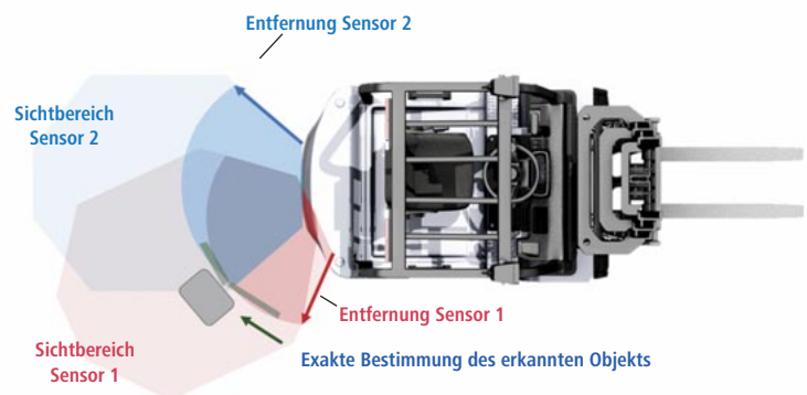
Zwei am Heck montierte Ultraschallsensoren (Foto oben) detektieren den rückwärtigen Nahbereich des Gabelstaplers. In der Detektionszone befindliche Objekte werden von den Sensoren erkannt (Grafik Draufsicht Gabelstapler von oben).
