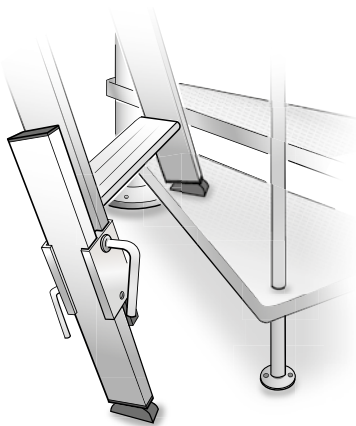
Abbildung 1: Holmverlängerung
